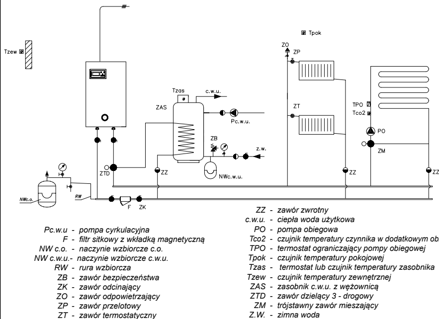
Rys.3 Przykładowa instalacja c.o. – grzejniki, ogrzewanie podłogowe, zasobnik, obieg c.w.u.
