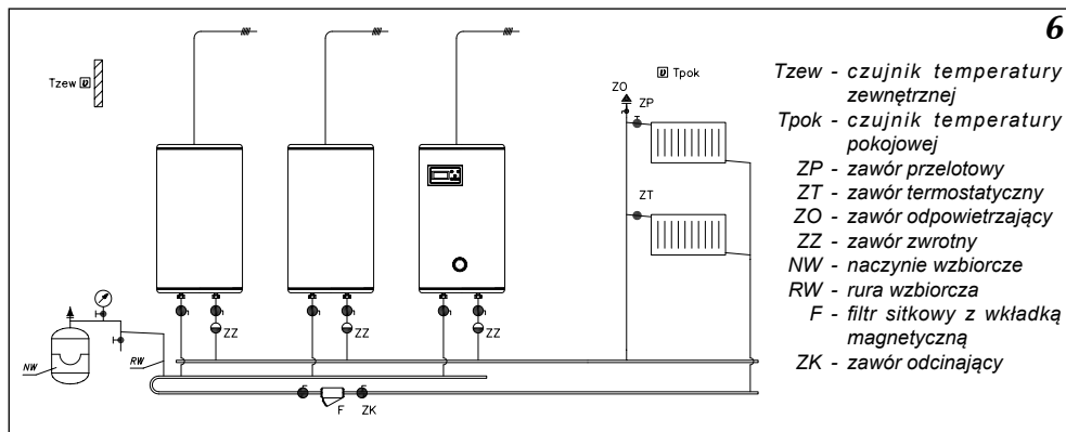
Rys.6 Połączenie grupy kotłów w sieć.
