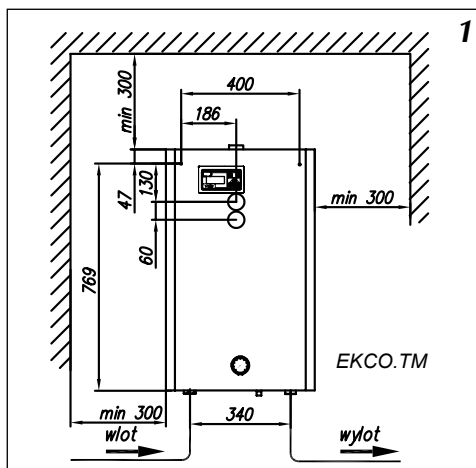
Rys.1 Sposób zamontowania kotła na ścianie.
