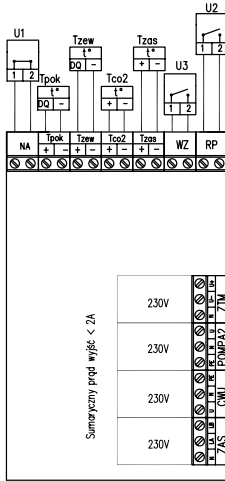
Rys.5 Podłączenie urządzeń zewnętrznych do modułu ZIO
